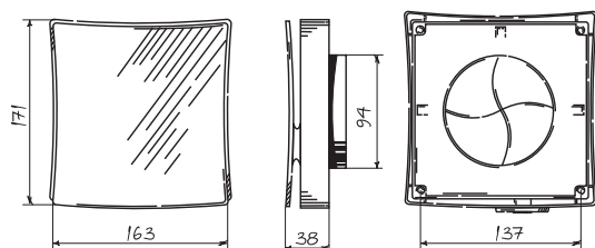
Наружная квадратная решетка (пластик)
