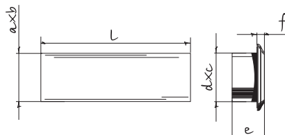
Прямоугольный ПВХ-воздуховод
